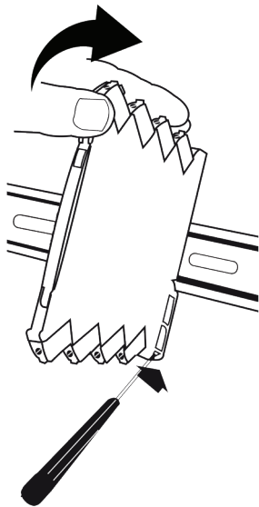
Imagen 2: Desmontaje del carril DIN. Primero, recuerde desmontar los conectores con tensiones peligrosas. Desconecte el dispositivo del carril DIN levantando la cerradura inferior.
