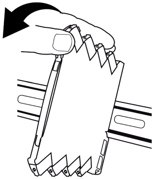
Imagen 1: Montaje en carril DIN. Haga clic en el dispositivo en el carril.
